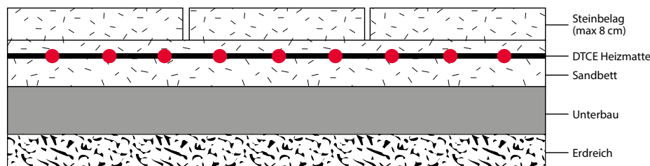
Freiflächenheizung mit Stein- oder Plattenbelag
