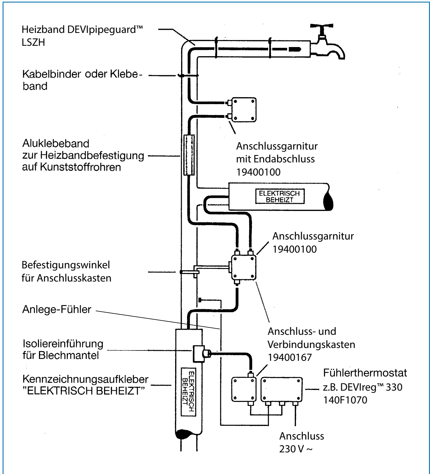
Montagebeispiel
