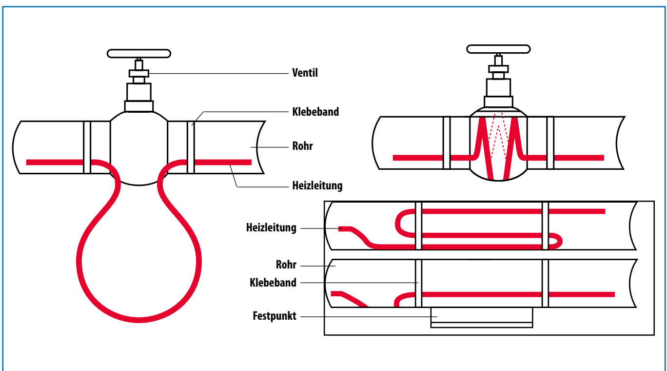
Installation an Ventilen und Flanschen
