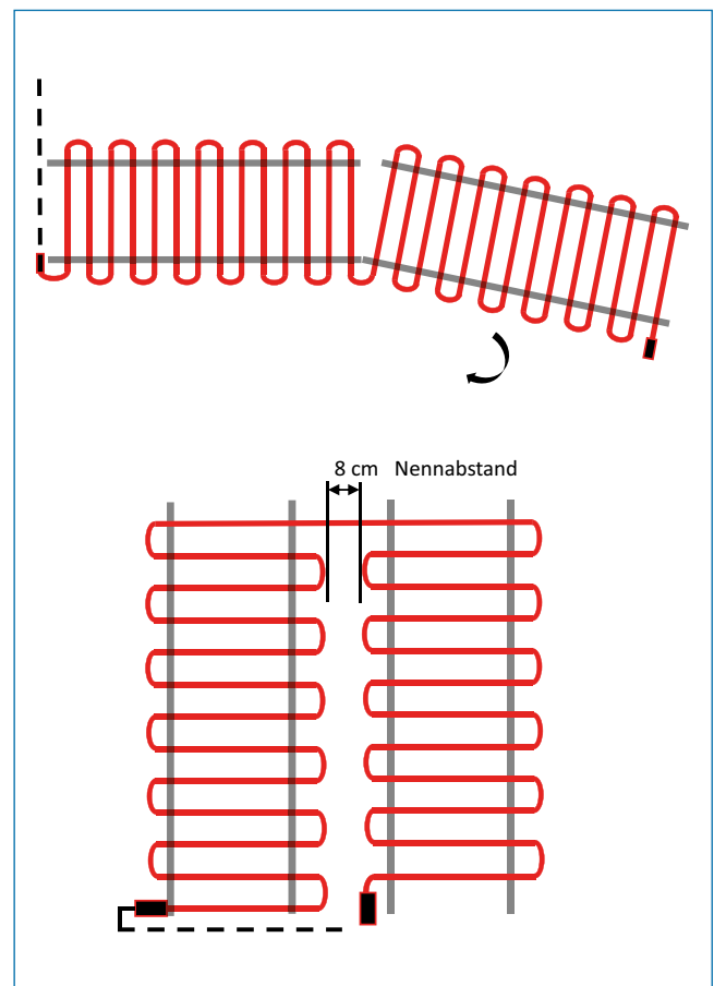
DEVImat™ (DTCE) montagefertige Heizmatte
