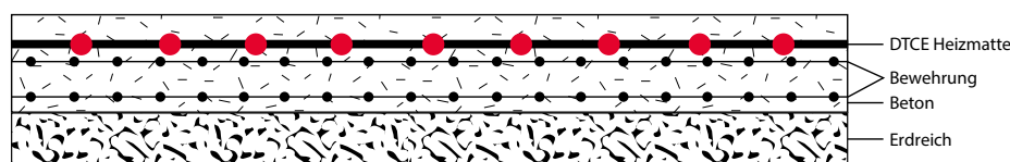
Beheizte Betonfläche
