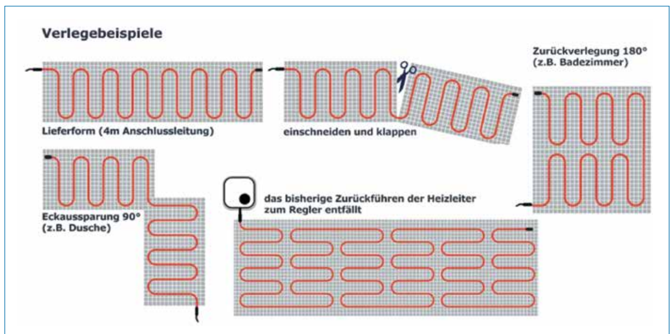
Verlegebeispiele
