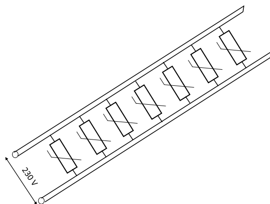
Ersatzschaltbild
