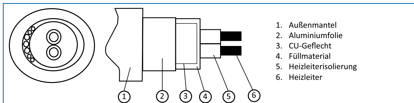
Aufbau einer DEVIsnow™ 20/30 (DTCE) Zweileiter Heizleitung
