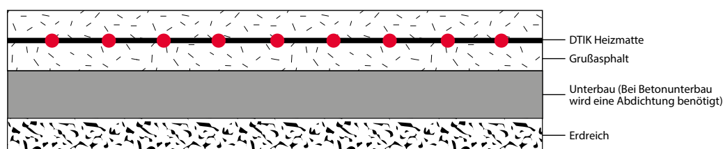
Freiflächenheizung mit Gußasphaltpelag
