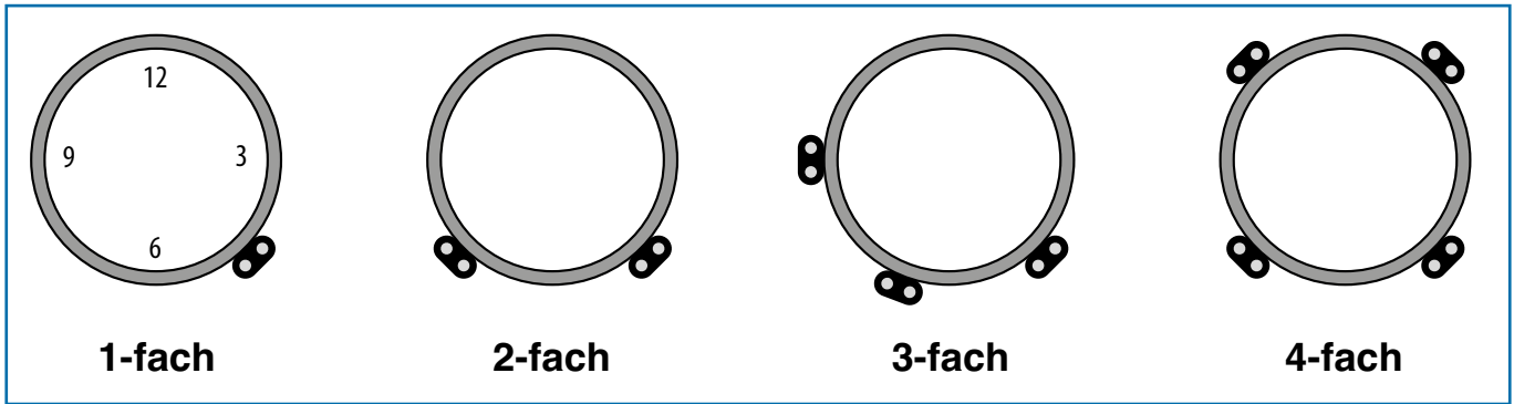
Einfach, zweifach, dreifach und vierfach Installation
