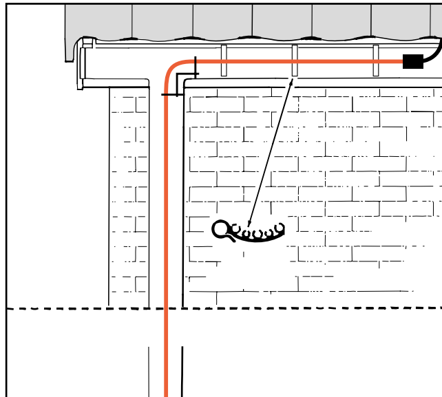
Fallrohr Ausführung
