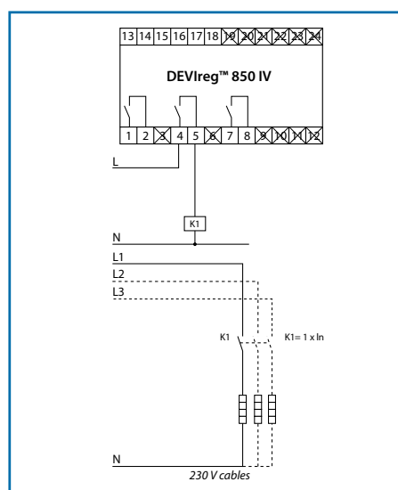
230 V direkter Anschluss Freifläche
