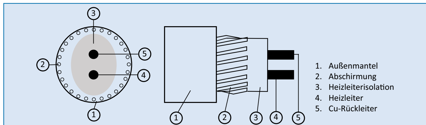
Aufbau einer Zweileiter-Heizleitung DTIP-10
