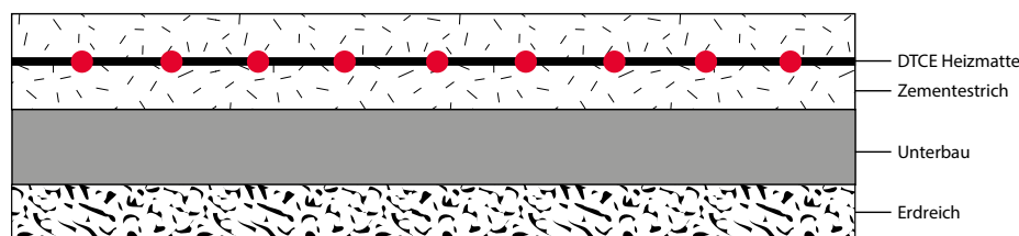
Freiflächenheizung im Estrich verlegt
